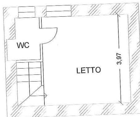
PIANO TERRA_scala 1:100
